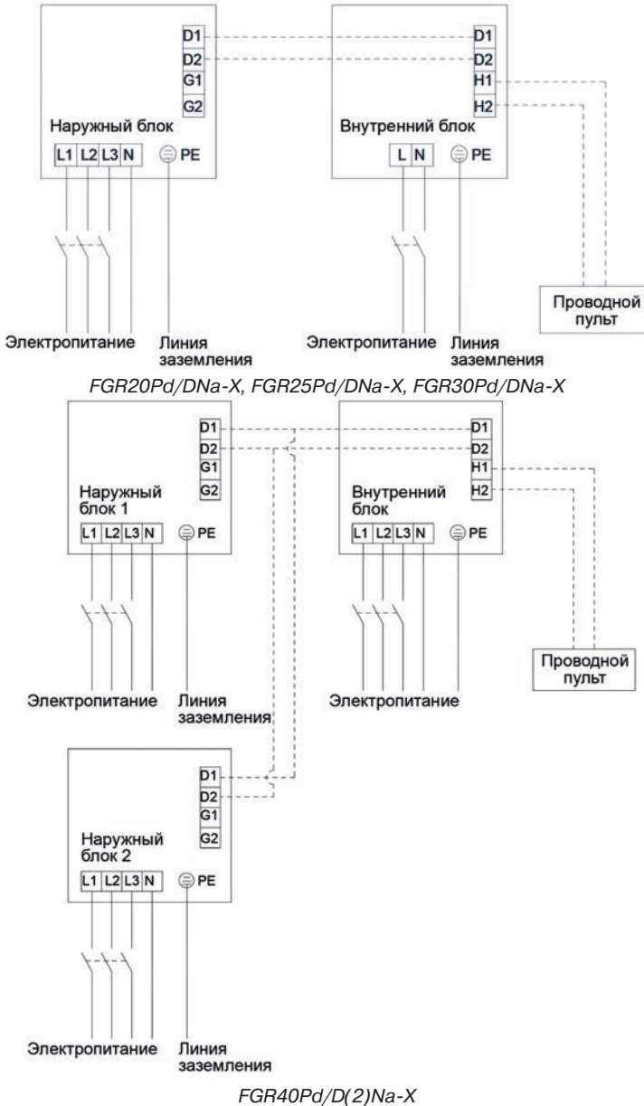
Рис. 22: Подключение силового и сигнального кабелей к внутреннему и наружному блокам.
