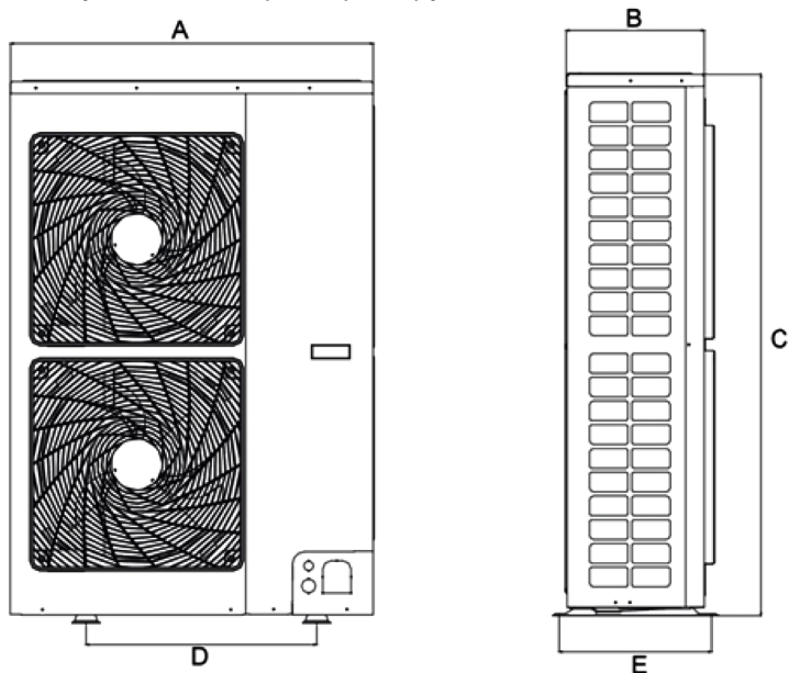
Рис. 16: Габаритные и установочные размеры наружного блока.
